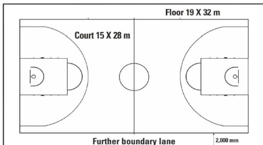
Рисунок 2 Майданчик та ігровий настил
